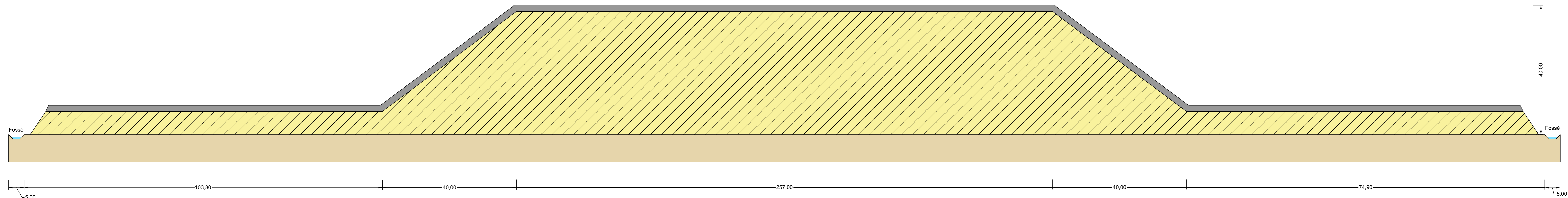
COUPE AB - BUTTE N°1
