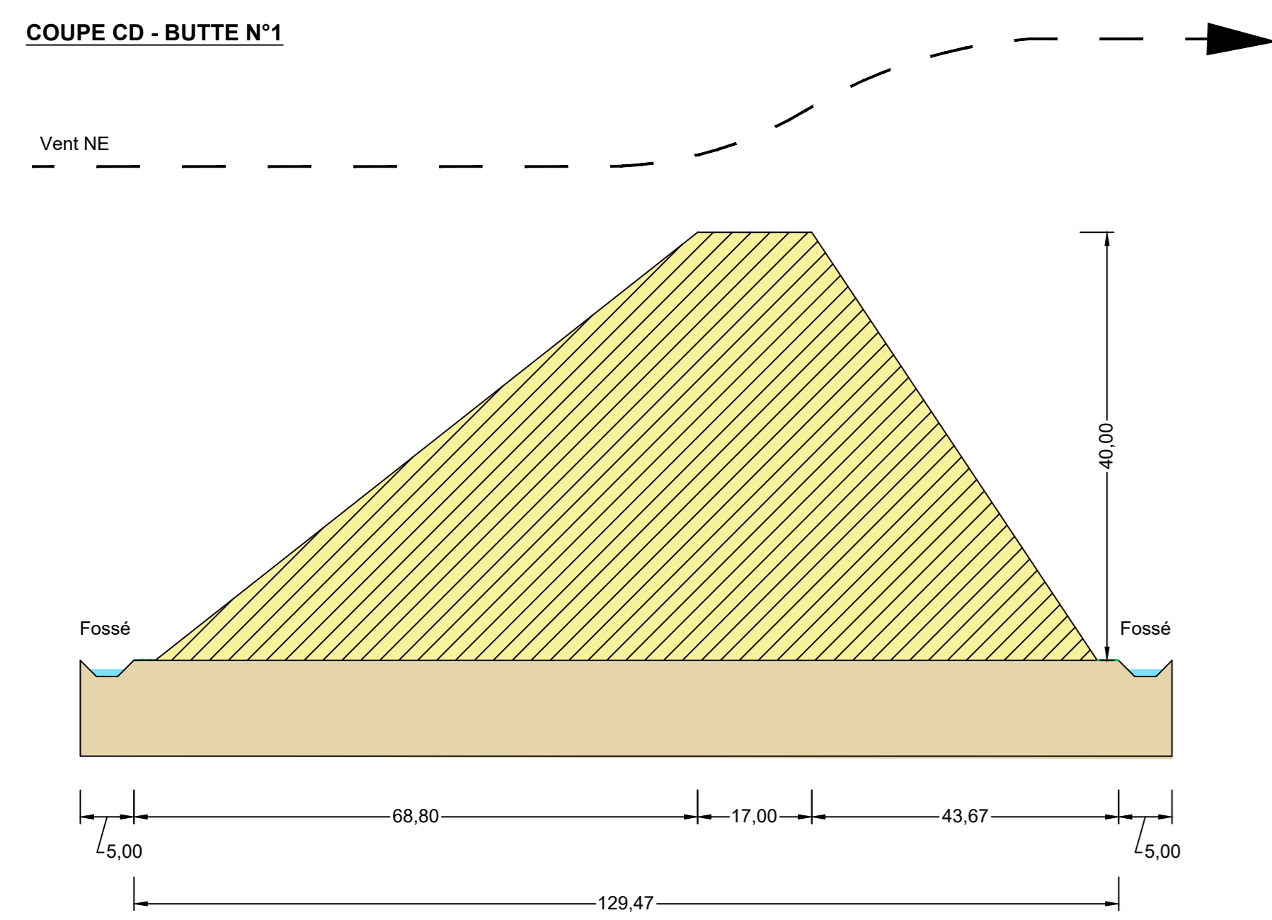
COUPE CD - BUTTE N°1
